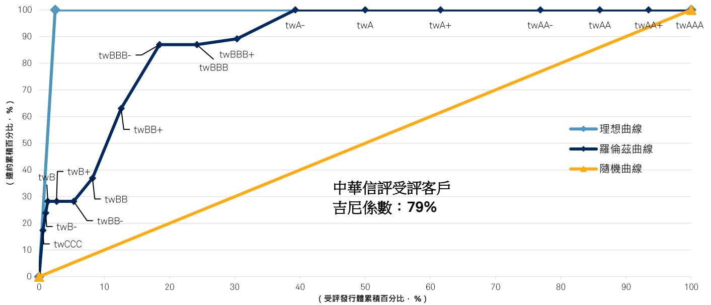
圖 4 中華信評受評企業五年期羅倫茲曲線與吉尼係數
